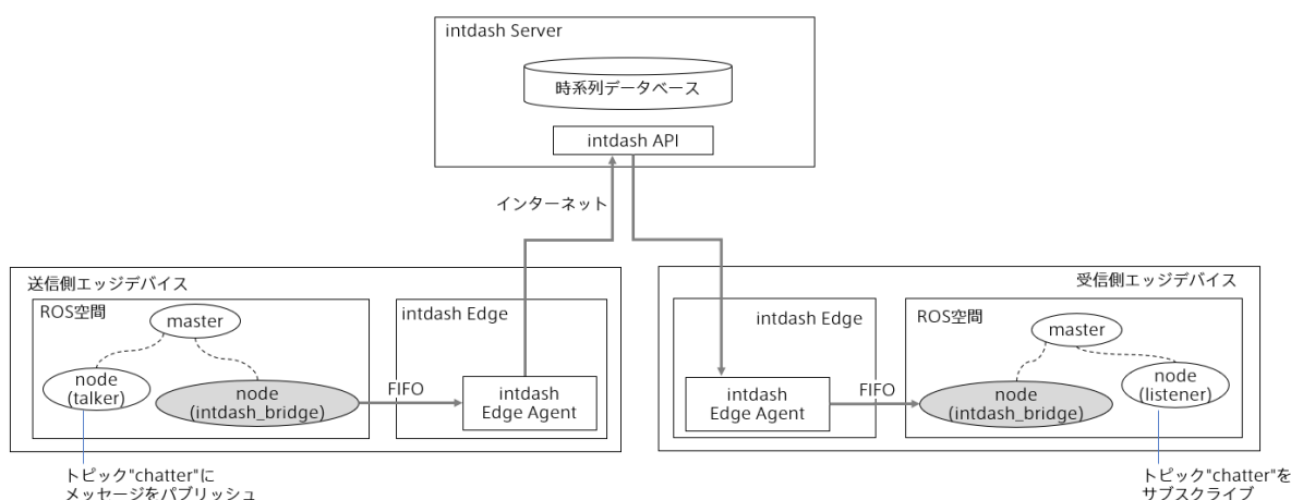
図 2 2 つの ROS 空間を接続する
