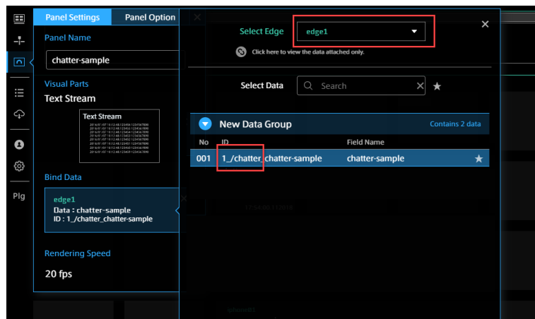
図 9 送信側エッジを選択し、パース設定を選択する
