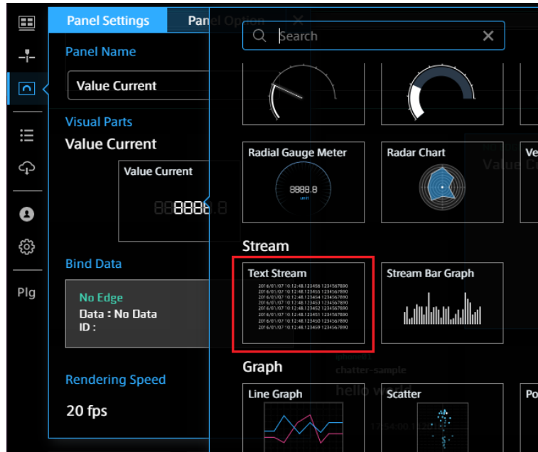
図 8 Text Stream
